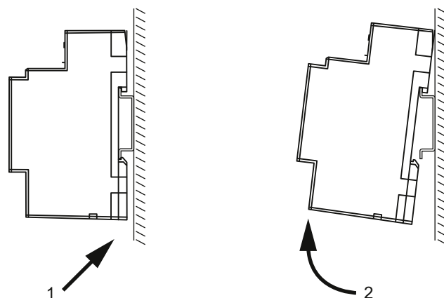
Fig. 16: Retirer le produit hors du rail
