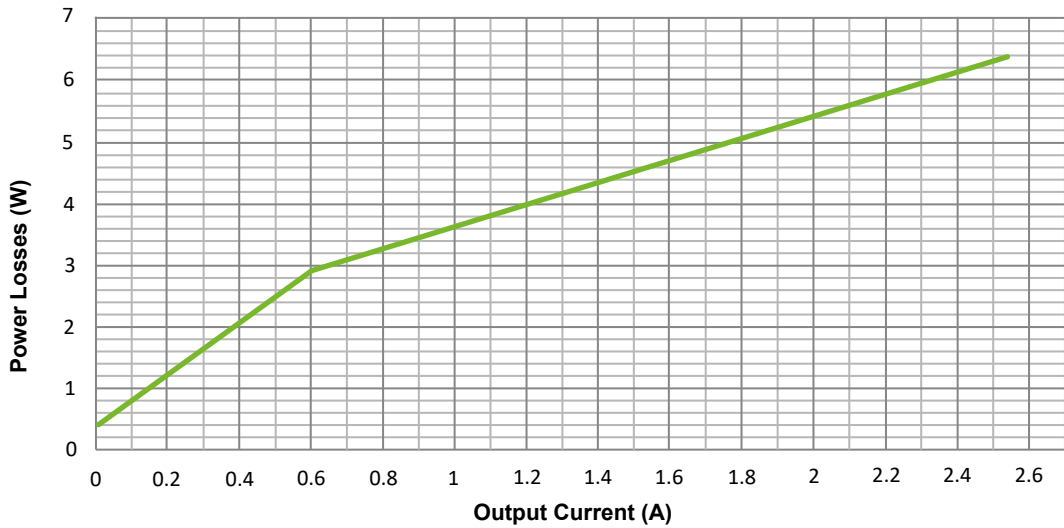
Fig. 12: Puissance dissipée pour 230 V AC
