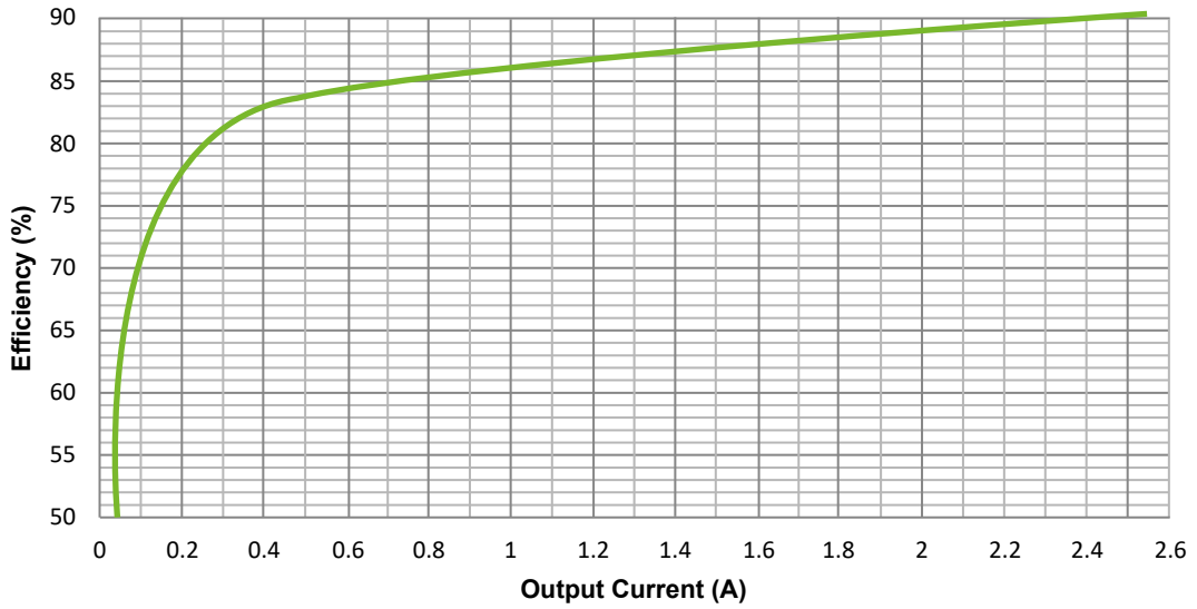
Fig. 11: Rendement pour 230 V AC
