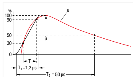
Spannungsimpuls 1,2/50 µs gemäß EN 60060-1/VDE 0432-1
