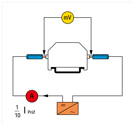
Prüfaufbau „Spannungsfallmessung“
