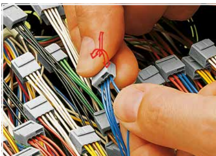
Lösen: Leiter festhalten, Klemme durch Hin- und Herdrehen mit leichtem Zug vom Leiter ziehen.
