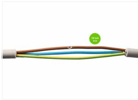
Beschädigte Leitung ca. 10 cm symmetrisch um die Schadstelle herum abmanteln.
