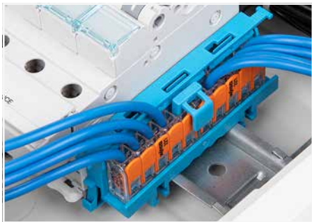
Mit Verriegelungsfunktion: Der Brücker mit Verriegelungsfunktion ist in die Verbindungsklemmen hineinsteckt.
