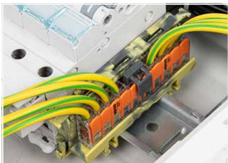
Der Brücker mit Verriegelungsfunktion ist in die Verbindungsklemmen hineinsteckt.
