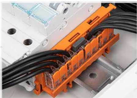
Ohne Verriegelungsfunktion: Der Brücker ohne Verriegelungsfunktion ist in die Verbindungsklemmen hineinsteckt.
