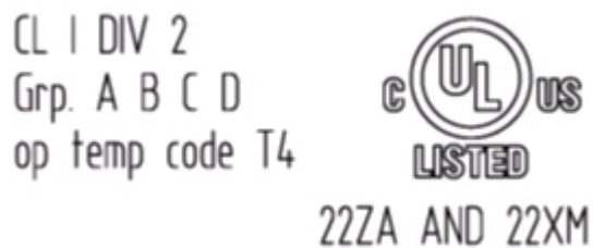
Abbildung 26: Textdetail - Beispielbedruckung der Busklemmen gemäß NEC 500
