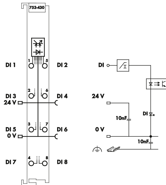
Abbildung 6: Schematisches Schaltbild
