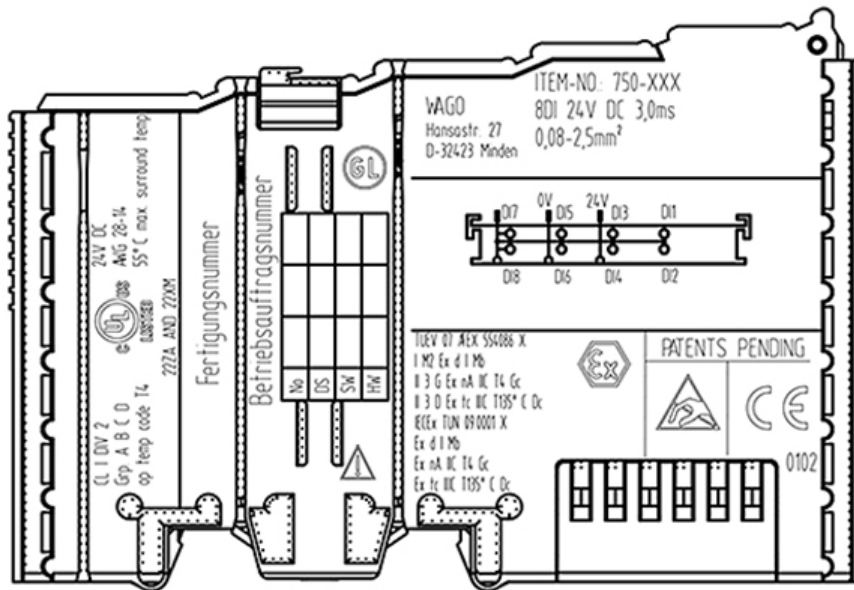
Abbildung 25: Beispiel für seitliche Bedruckung der Busklemmen gemäß NEC 500
