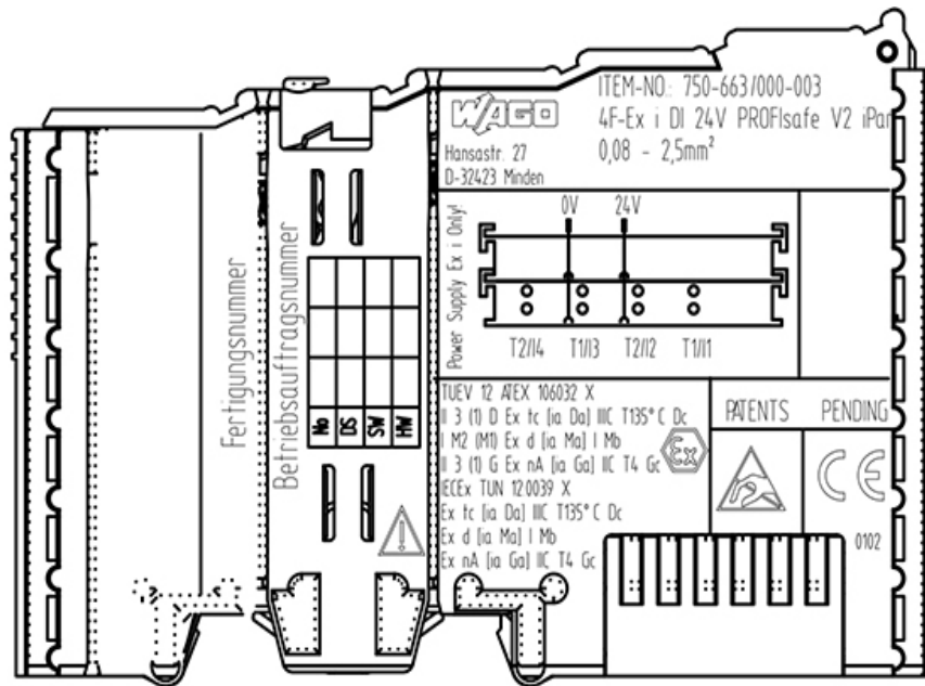
Abbildung 23: Beispiel für die seitliche Bedruckung der ATEX- und IECEx-zugelassenen Ex i Busklemmen.
