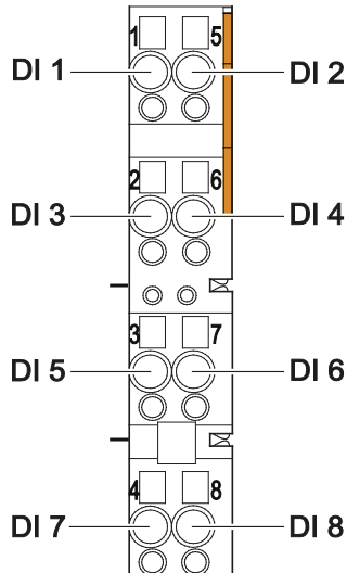
Abbildung 4: CAGE CLAMP®-Anschlüsse
