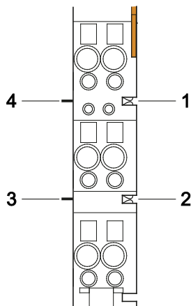
Abbildung 3: Leistungskontakte
