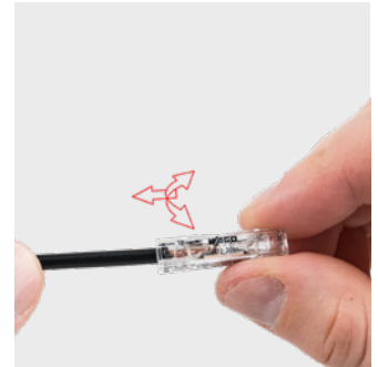
Lösen: Bei eindrätigen Leitern Klemme durch Hin- und Herdrehen mit leichtem Zug vom Leiter ziehen. Bei mehrdrätigen Leitern Ader abschneiden und neue Klemme verwenden.
