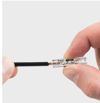
Anschließen: Abisolierten eindrätigen oder mehrdrätigen Leiter bis zum Anschlag einstecken.
