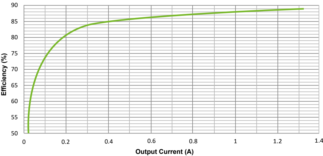
Fig. 11: Rendement pour 230 V AC
