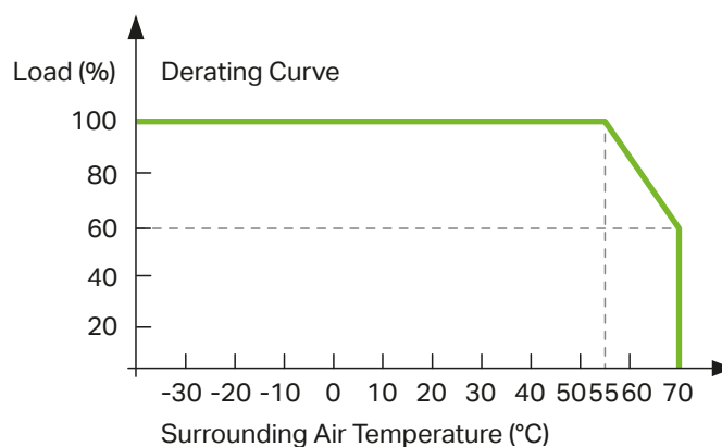
Fig. 13: Déclassement - Température ambiante
