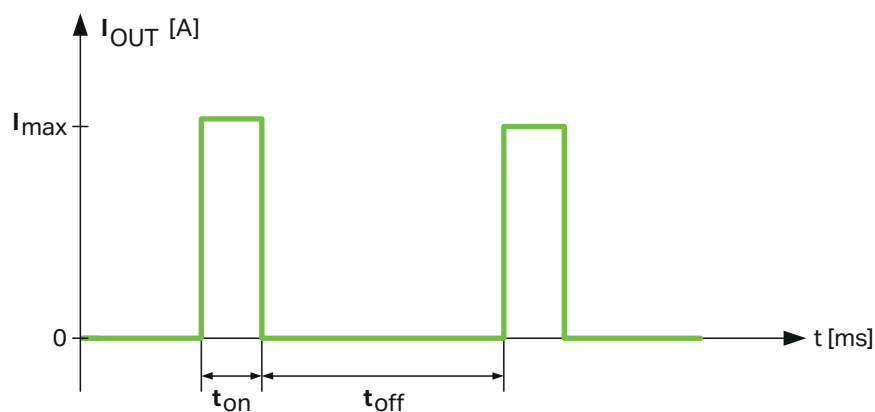
Fig. 9: Mode hiccup
