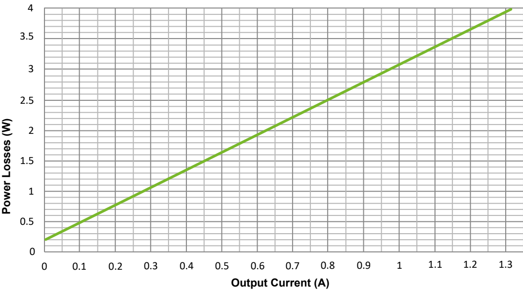
Fig. 12: Puissance dissipée pour 230 V AC
