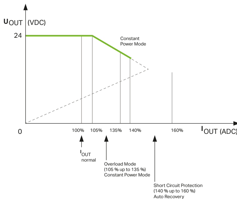
Fig. 22: Caractéristique de sortie
