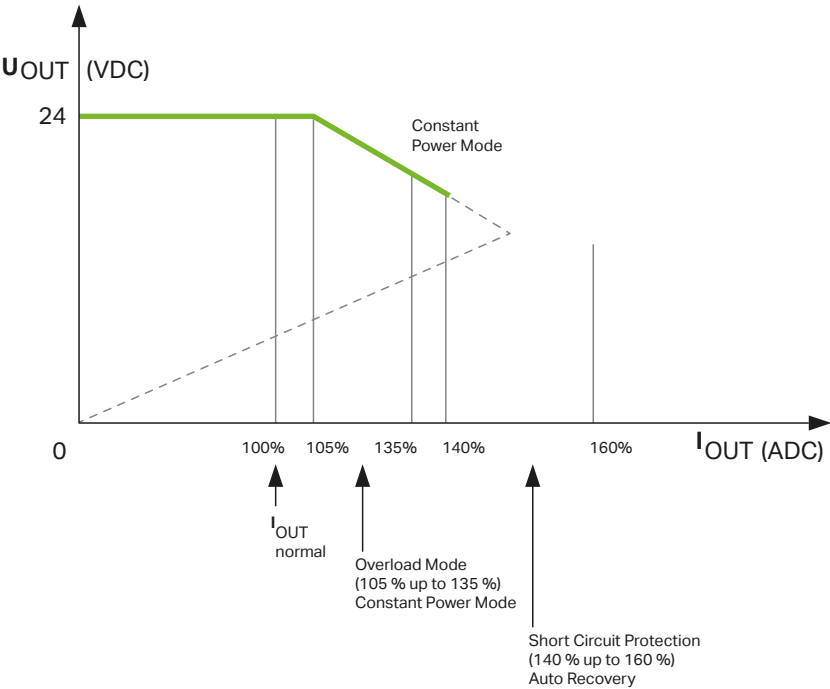
Fig. 8: Comportement en surcharge
