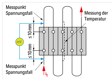
Prüfaufbau „Erwärmungsprüfung“
