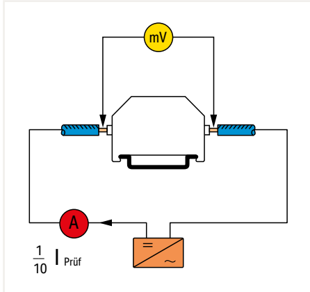
Prüfaufbau „Spannungsfallmessung“
