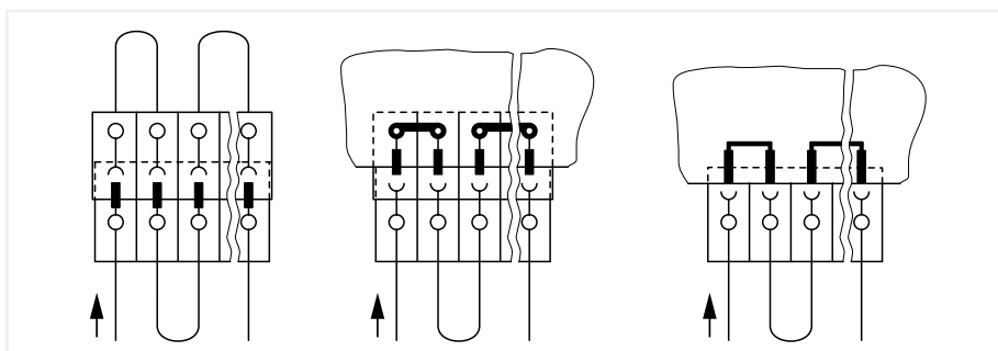
Prüfaufbau „Erwärmungsprüfung“ gemäß IEC/EN 61984
