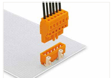
Stifteleiste mit geraden Einlötschäften Federleiste mit CAGE CLAMP®-Anschluss
