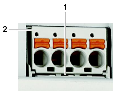
Ilustracja 10: Wyciąganie gniazda bez zamocowanych przewodów (przykład zastosowania)
