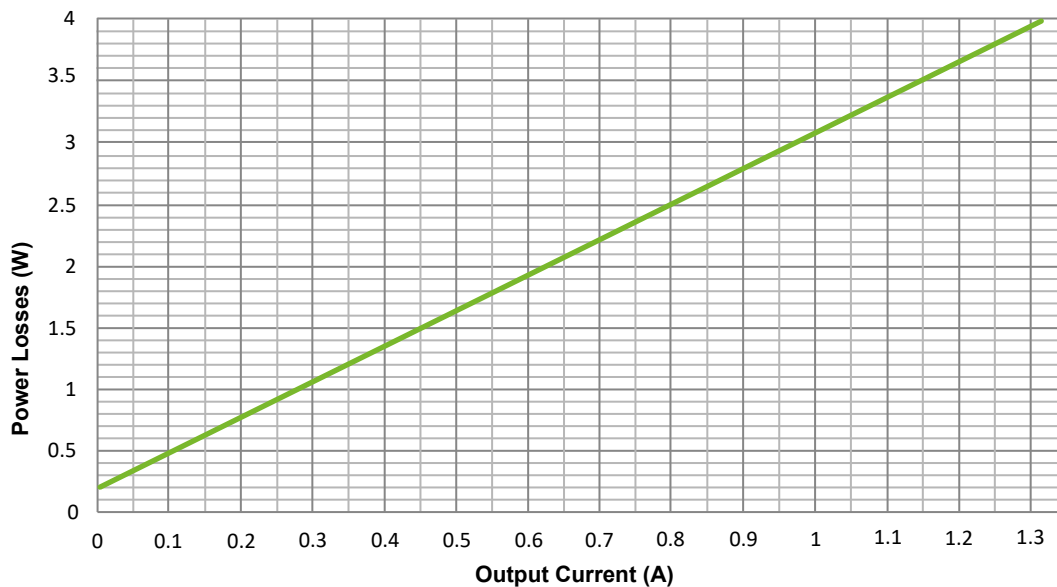
Рис. 12: Потеря мощности при 230 В перем. тока
