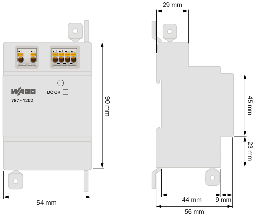
Рис. 7: Габаритные размеры
