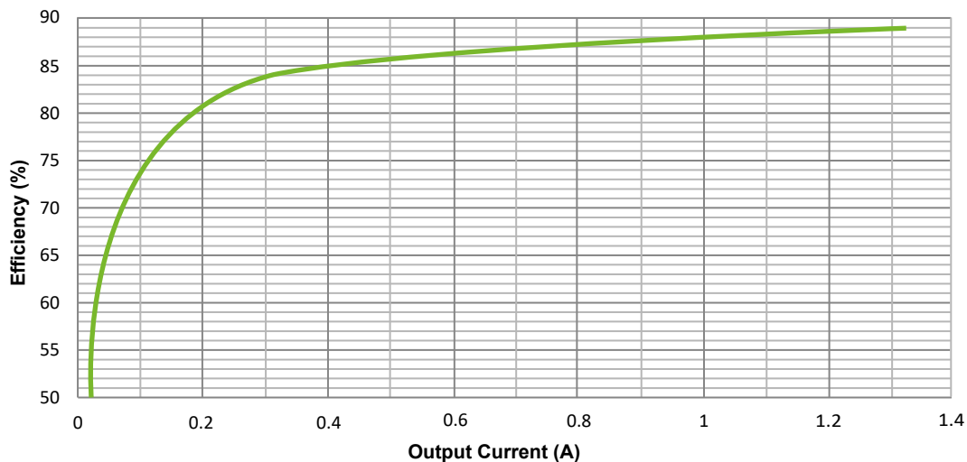
Рис. 11: Эффективность при 230 В перем. тока
