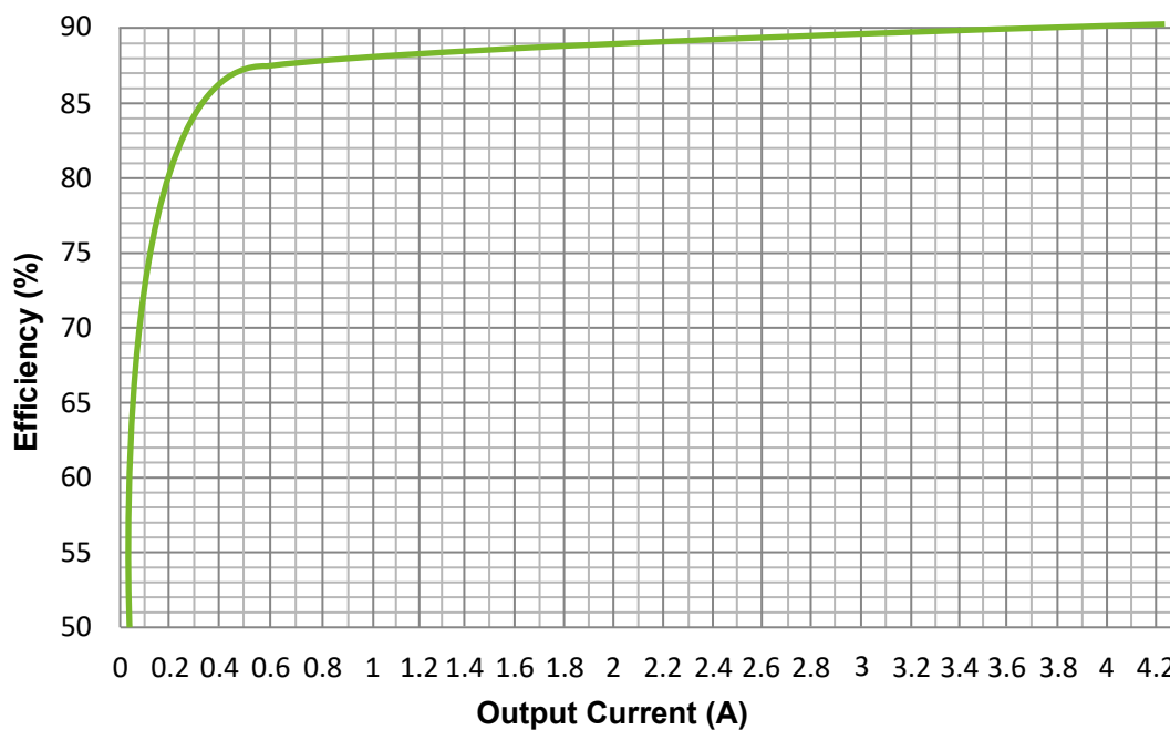
Fig. 11: Rendement pour 230 V AC
