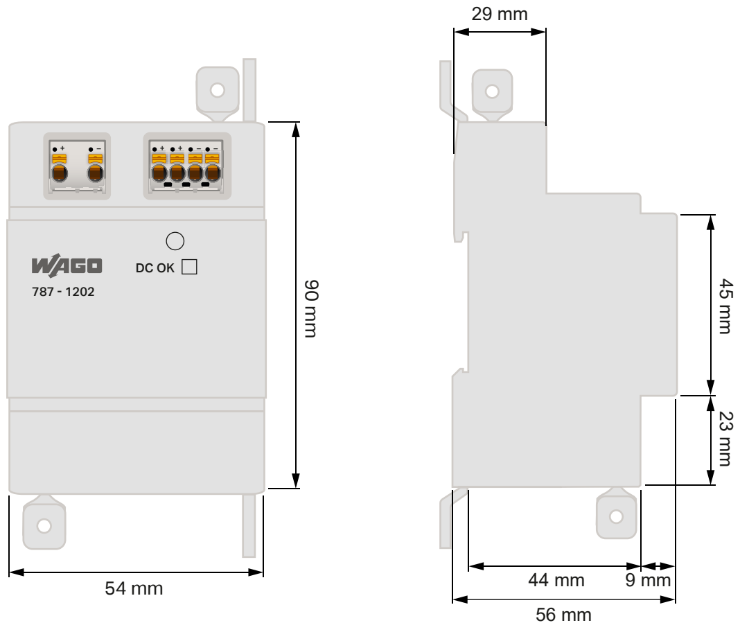
Abbildung 7: Abmessungen
