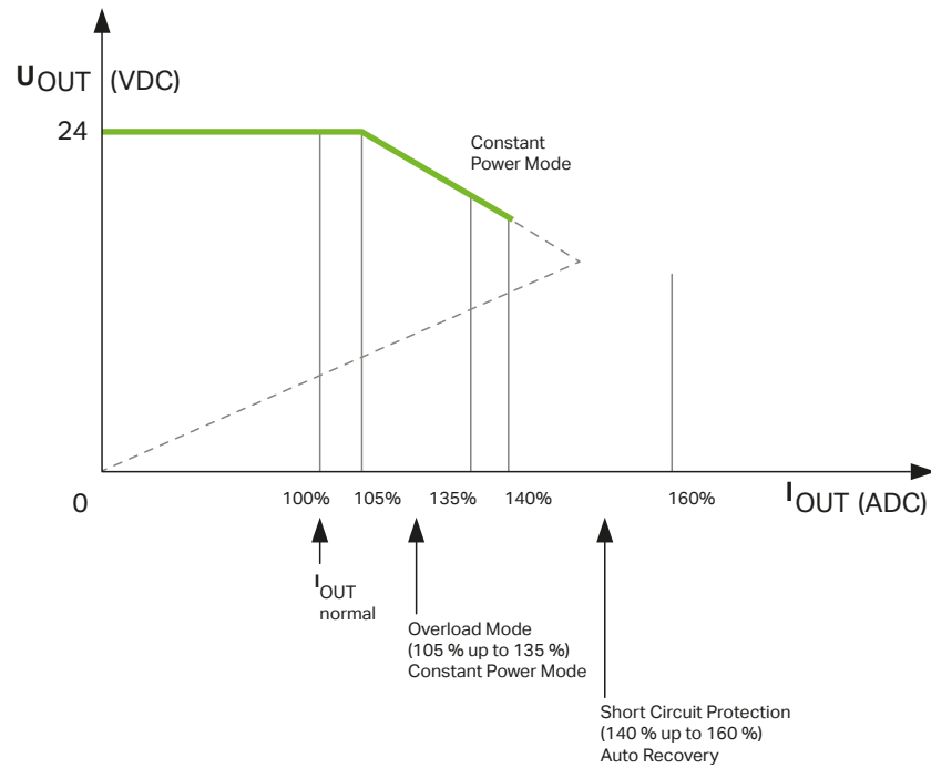
Abbildung 8: Überlastverhalten
