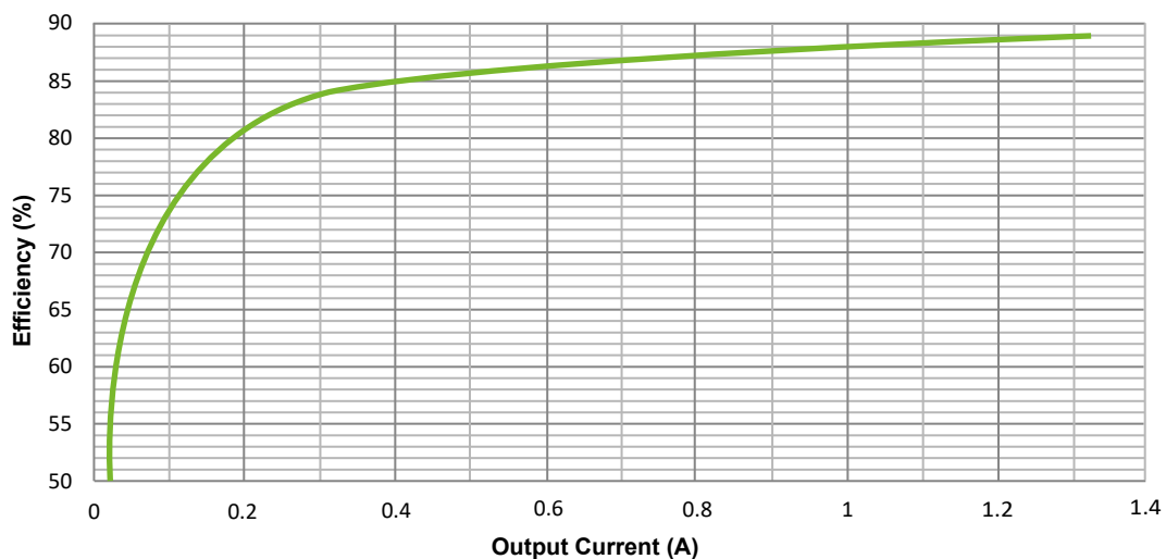
Abbildung 11: Wirkungsgrad bei AC 230 V
