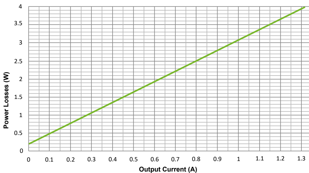
Abbildung 12: Verlustleistung bei AC 230 V
