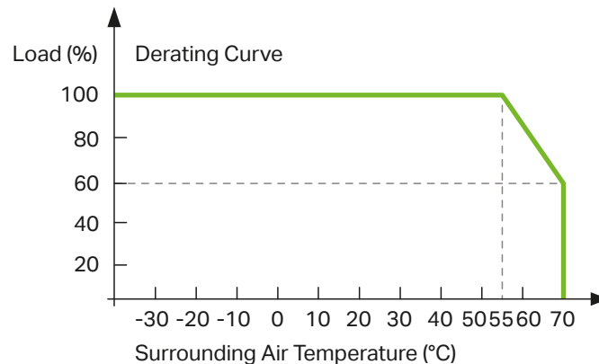
Abbildung 13: Derating-Umgebungstemperatur
