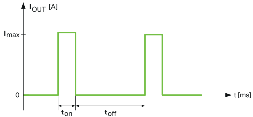
Abbildung 9: Hiccup-Mode
