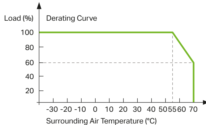
Abbildung 21: Temperaturlastkennlinie
