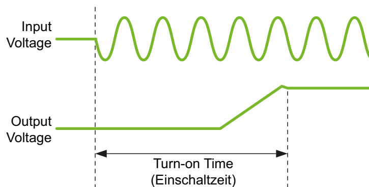
Abbildung 10: Einschaltzeit
