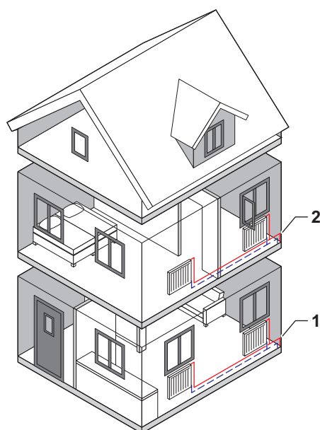
Abb.5 Zwei Heizkreise
