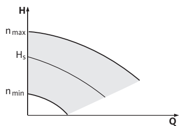
Fig. 43 : Mode régulation de vitesse
