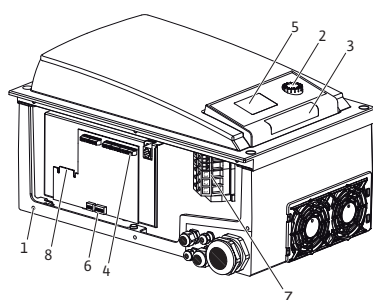
Fig. 9 : Module électronique
