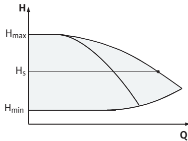
Fig. 14: Regelung Δp-c (Parallelbetrieb)
