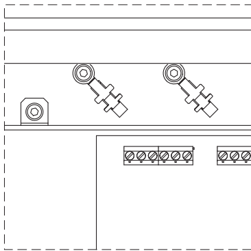
Fig. 23: Kabelabschirmung
