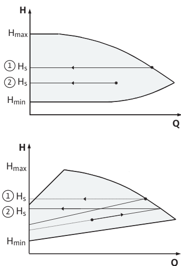
Fig. 42 : Régulation \Delta p\text{-}c/\Delta p\text{-}v
