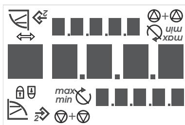
Fig. 30 : Test d'affichage
