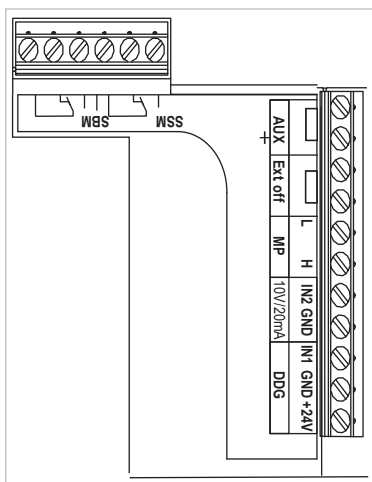
Fig. 24: Stuurklemmen
