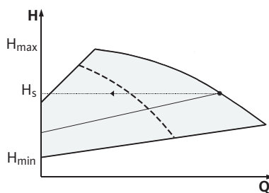
Fig. 15: Regelung Δp-v (Parallelbetrieb)
