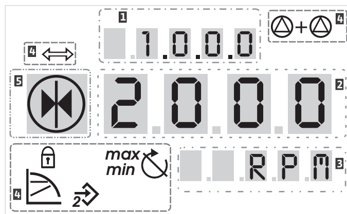
Fig. 29: Displayaufbau
