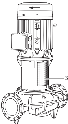
Fig. 8: Montiertes Kupplungsschutzblech
