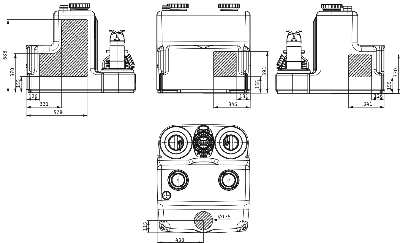
Fig. 4: Zulaufflächen
