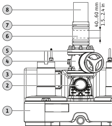
Fig. 3: Druckanschluss montieren
