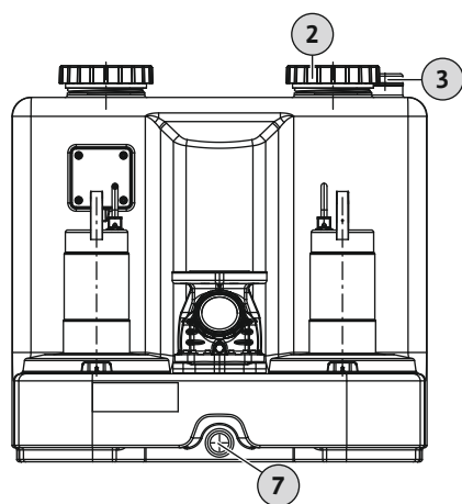
Fig. 7: Anschluss Handmembranpumpe
