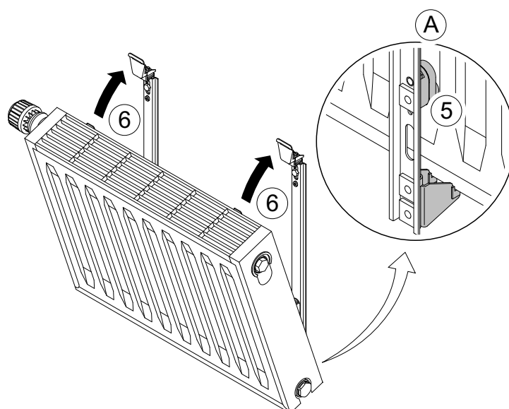
Abb. 4: Flachheizkörper einsetzen
