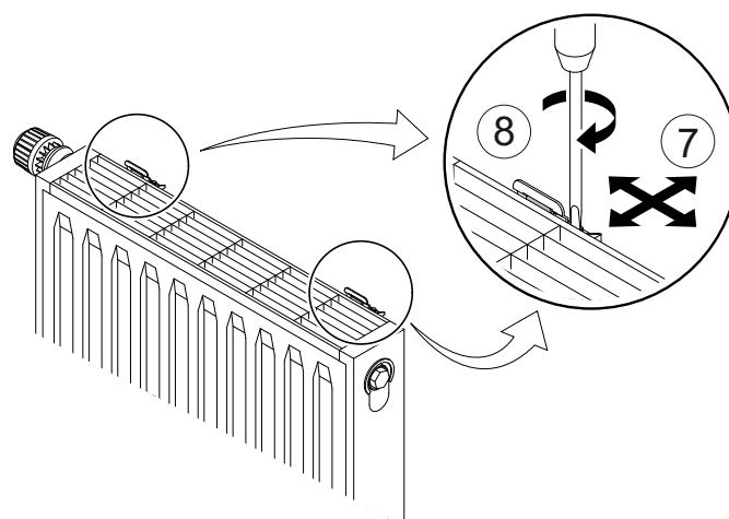
Abb. 5: Flachheizkörper ausrichten und befestigen
