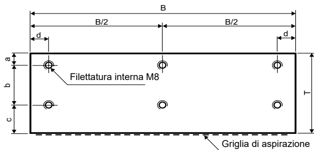
Vista dall'alto dell'apparecchio - fissaggio a soffitto
