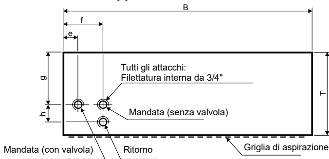
Vista dall'alto dell'apparecchio - attacco tubazione
