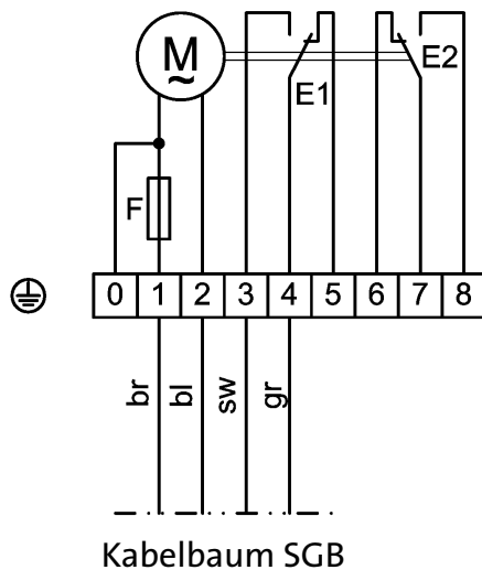
Abb 1: Schaltplan Zuluftklappe alt - Stellantrieb STA 2 EW
