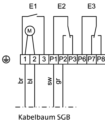
Abb 2: Schaltplan Zuluftklappe neu - Stellantrieb STA 2 (S3)
